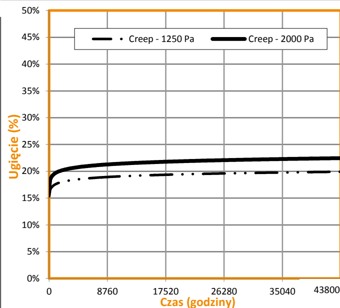
Pełzanie materiału - EN 1606 (4)
